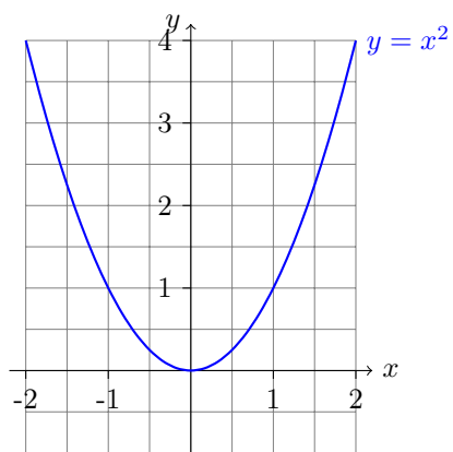
Σχήμα 1: Συνάρτηση y = x^2
