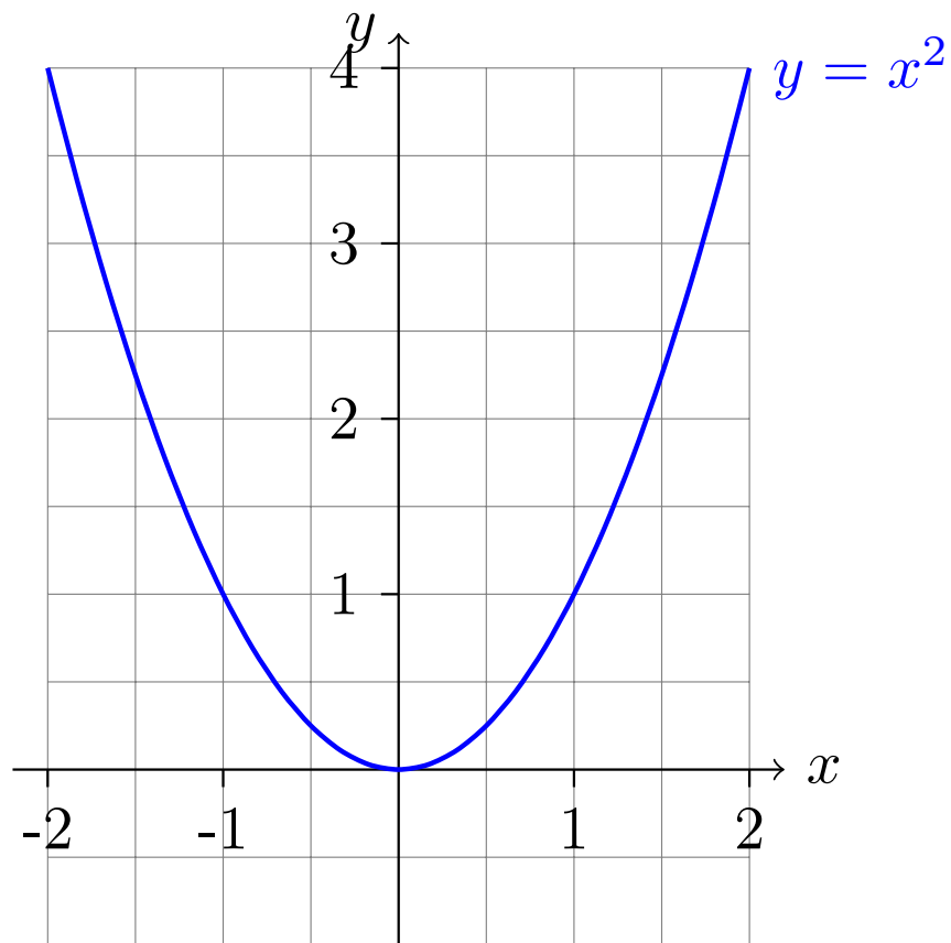
Σχήμα 1: Συναρτηση y = x^2
