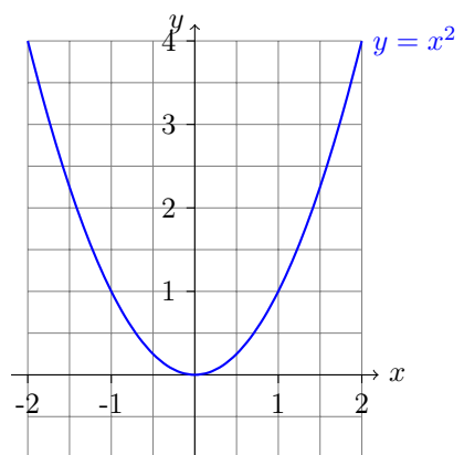
Σχήμα 1: Συνάρτηση y = x^2
