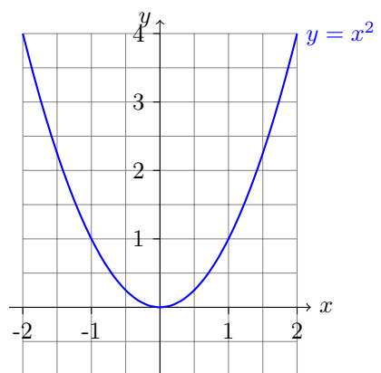
Σχήμα 1: σφναρτηση y = x^2
