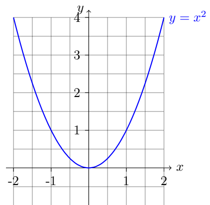
Σχήμα 1: ΣΥΝΑΡΤΗΣΗ y = x^2
